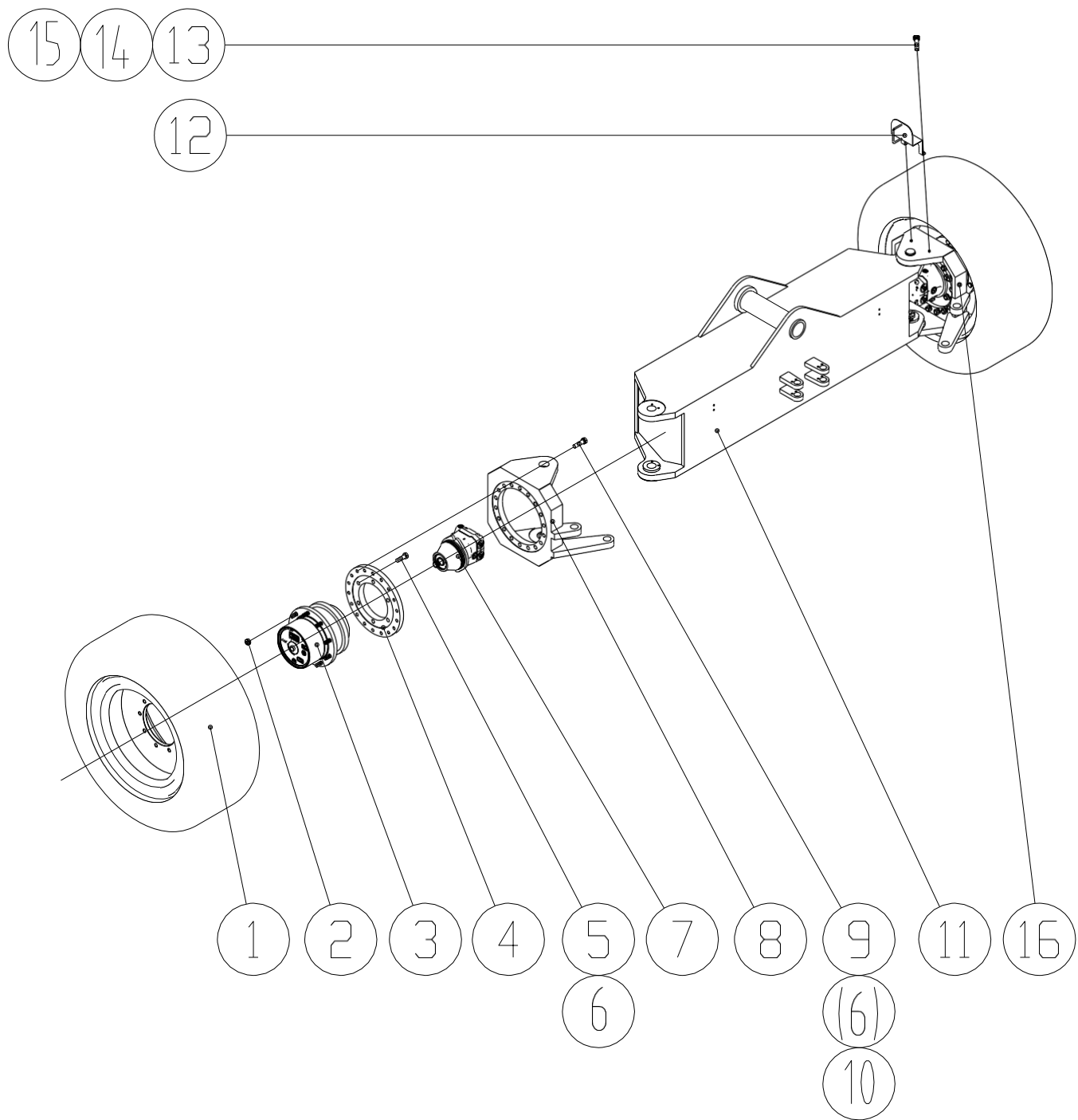
图号 (Figure) 描述 (Description) 202. 2 HZ280H 方向盘轴和轮胎
